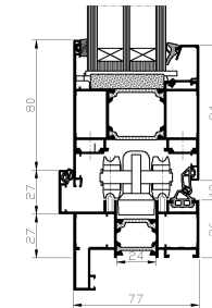
Przekrój: 13, 33 wariant 4
