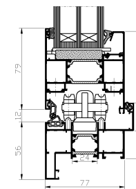
Przekrój: 13, 33 wariant 5
