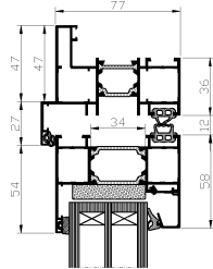
Przekrój: 12, 32 wariant 3
