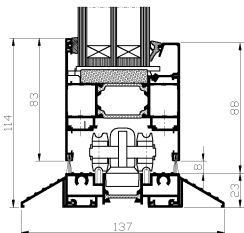
Przekrój: 13, 33 wariant 13
