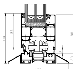
Przekrój: 13, 33 wariant 14
