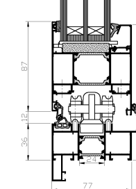
Przekrój: 13, 33 wariant 6
