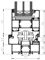
Przekrój: 13, 33 wariant 1
