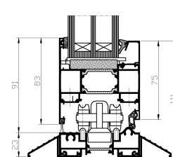
Przekrój: 13, 33 wariant 10
