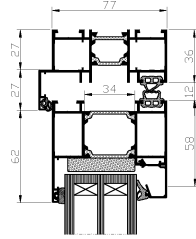
Przekrój: 12, 32 wariant 2
