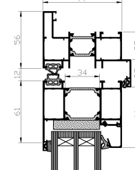
Przekrój: 12, 32 wariant 6
