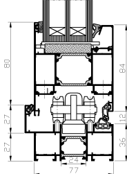
Przekrój: 13, 33 wariant 2
