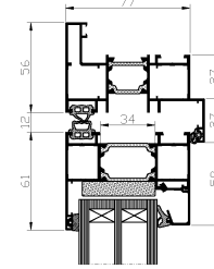
Przekrój: 12, 32 wariant 5
