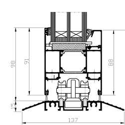
Przekrój: 13, 33 wariant 11
