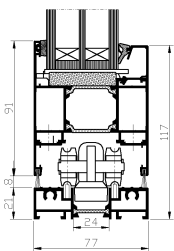
Przekrój: 13, 33 wariant 7
