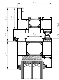
Przekrój: 12, 32 wariant 4
