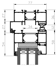
Przekrój: 12, 32 wariant 1
