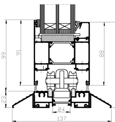
Przekrój: 13, 33 wariant 9
