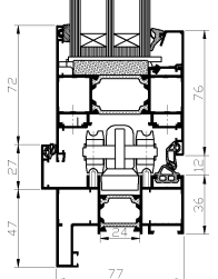
Przekrój: 13, 33 wariant 3
