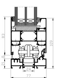
Przekrój: 13, 33 wariant 8
