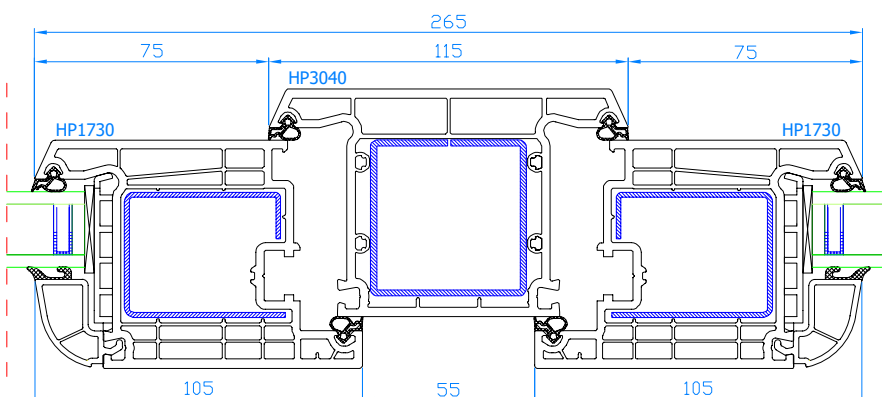
DPB-73 Meneau fixe Vaste middenstijl
