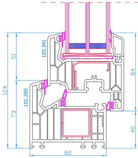
DPQ-82 Ouvrant standard Standaard vleugel
