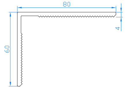
Cornière 80x60 Afdekprofiel 80x60
