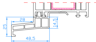
Seuil 28x48,5 Vensterbankdorpel 28x48,5
