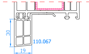
Aile rapportée 30x19 Vensterbanklijst 30x19
