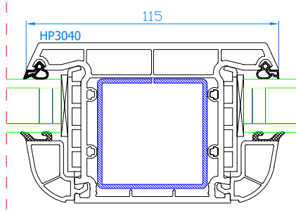
DPB-73 Meneau fixe Vaste middenstijl
