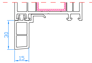
Aile rapportée 30x15 Vensterbanklijst 30x15
