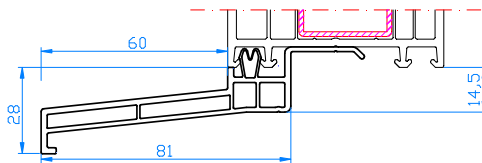
Piece d'appui 60x81 Vensterbankdorpel 60x81
