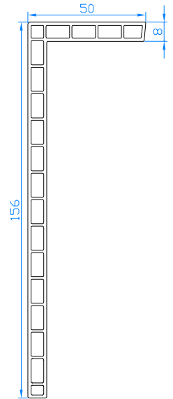
Cornière 50x156 Afdekprofiel 50x156
