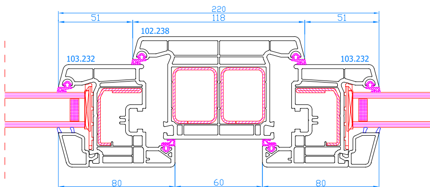
DPP-70 Meneau fixe Vaste middenstijl
