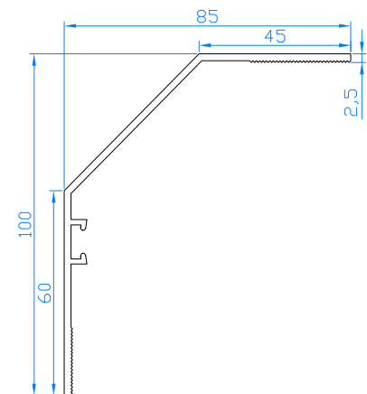
Cornière pan coupe 85x100 Afdekprofiel 85x100
