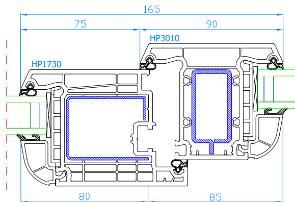
DPB-73 Meneau fixe Vaste middenstijl
