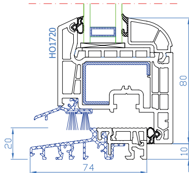
DPB-73 Porte-fenêtre avec seuil plat alu Balkondeur met lage alu-dorpel
