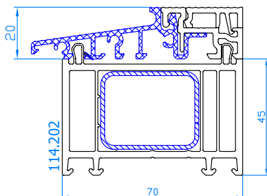
Élargisseur pour seuil plat alu (TS58212) Verbreding 45 mm voor alu-dorpel
