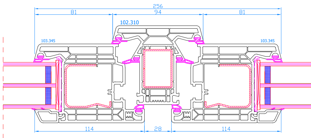
DPQ-82 Meneau fixe Vaste middenstijl
