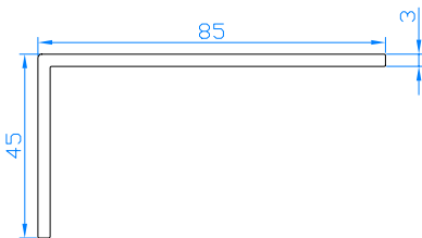
Cornière 85x45 Afdekprofiel 85x45
