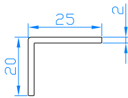
Cornière 25x20 Afdekprofiel 25x20
