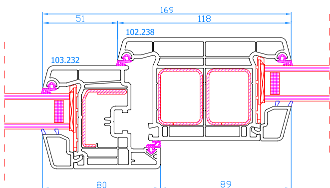
DPP-70 Meneau fixe Vaste middenstijl
