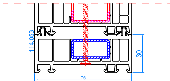
Élargisseur 30 mm Verbreding 30 mm
