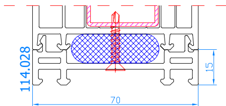
Élargisseur 15 mm Verbreding 15 mm
