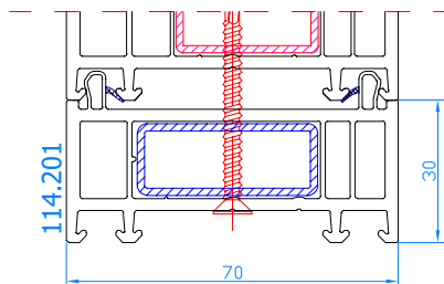
Élargisseur 30 mm Verbreding 30 mm
