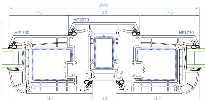
DPB-73 Meneau fixe Vaste middenstijl
