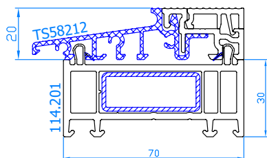
Élargisseur pour seuil plat alu (TS58212) Verbreding 30 mm voor alu-dorpel
