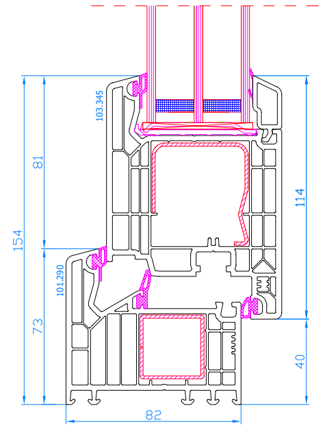
DPQ-82 Ouvrant large Brede vleugel
