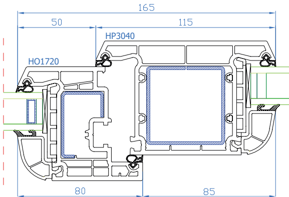
DPB-73 Meneau fixe Vaste middenstijl
