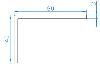
Cornière 60x40 Afdekprofiel 60x40
