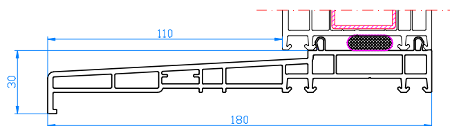
Piece d'appui 20x180 Vensterbankdorpel 20x180
