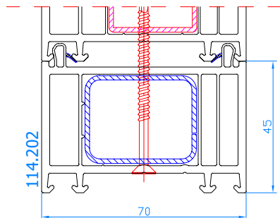
Élargisseur 45 mm Verbreding 45 mm
