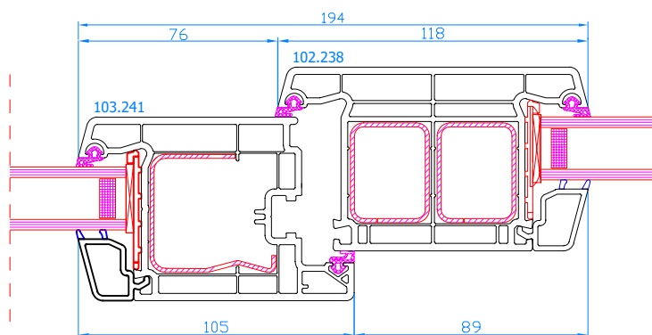
DPP-70 Meneau fixe Vaste middenstijl
