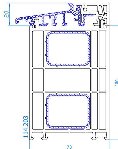
Élargisseur pour seuil plat alu (TS58212) Verbreding 100 mm voor alu-dorpel
