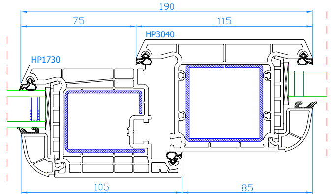
DPB-73 Meneau fixe Vaste middenstijl
