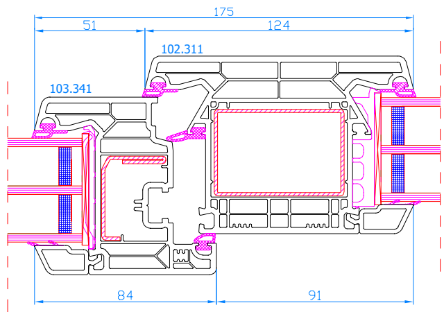
DPQ-82 Meneau fixe Vaste middenstijl
