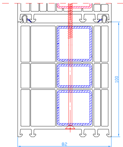
Élargisseur 100 mm Verbreding 100 mm
