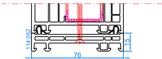
Élargisseur 15 mm Verbreding 15 mm
