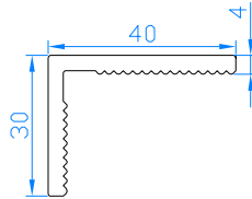
Cornière 40x30 Afdekprofiel 40x30
