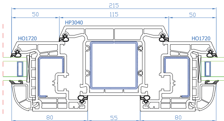
DPB-73 Meneau fixe Vaste middenstijl
