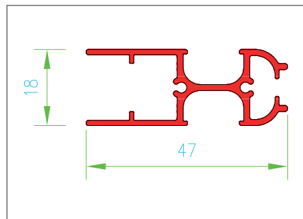
Rys. 8 Posuvný ouzký profil
