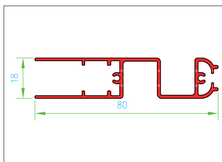
Rys. 2 Standardní posuvný profil
