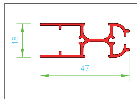
Rys. 3 Posuvný ouzký profil
