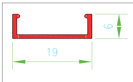
Rys. 5 Spodní plochý profil
