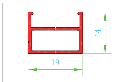
Rys. 4 Dolní standardní profil
