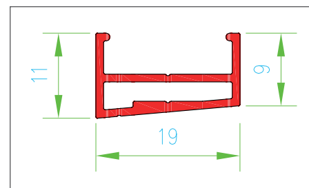
Rys. 6 Svažující spodní profil
