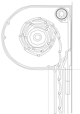
VORBAUSYSTEM DK-RZO integriertes Insektenschutzgitter
