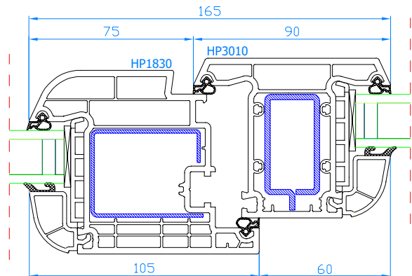
DPB-73+ Setzpfosten Setzpfosten: HP3010 breiter Flügel: HP1830
