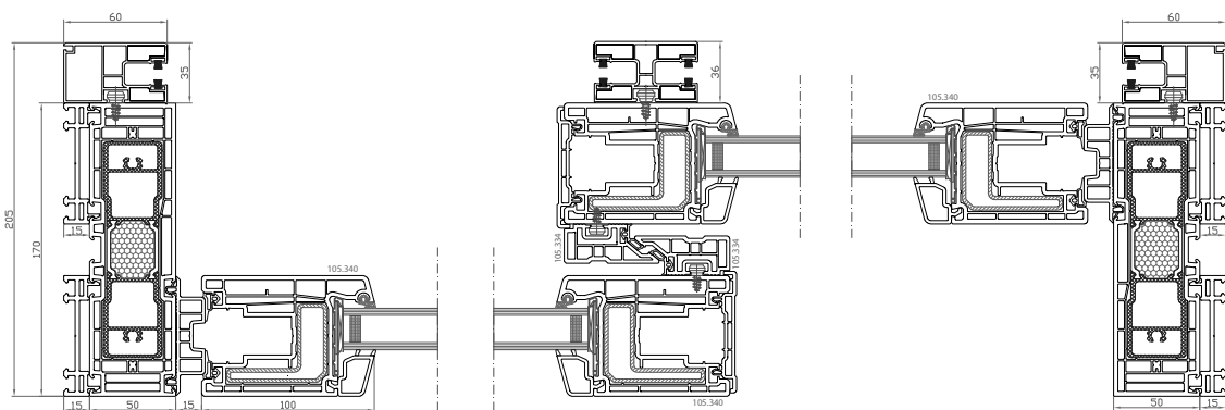
DPP-70 HST Aufsatzrollläden: DK-RNB Draufsicht
