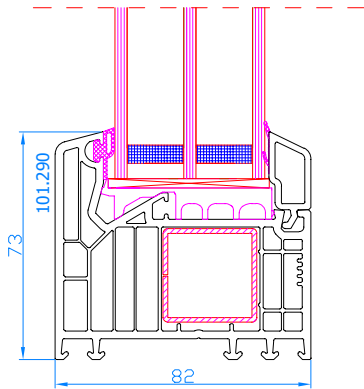
DPQ-82 Festverglasung im Rahmen Rahmen: 101.290
