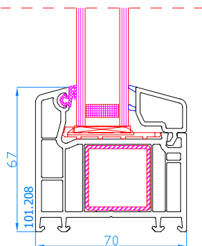
DPP-70 Festverglasung im Rahmen Rahmen: 101.208
