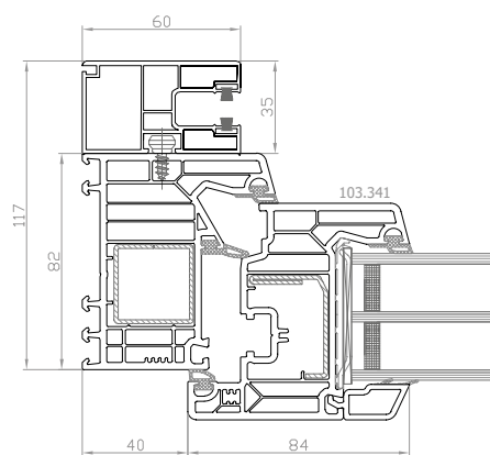
DPQ-82 Draufsicht
