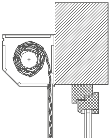
DK-RZS vorne an der Wand montiert
