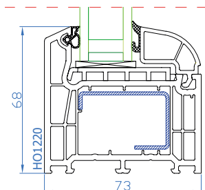
DPB-73 Festverglasung im Rahmen Rahmen: HO1220
