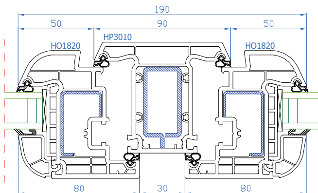
DPB-73+ Setzpfosten Setzpfosten: HP3010 Flügel: HO1820
