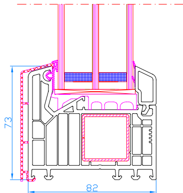
DPQ-82 AL Festverglasung im Rahmen Rahmen: 101.290
