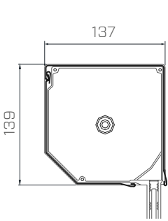
DK-RZS Kasten 137
