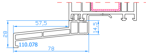
Fensterbankanschlußprofil 28x78 Code: 110.078
