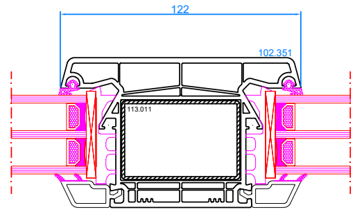
DPQ-76 Setzpfosten Setzpfosten: 102.351
