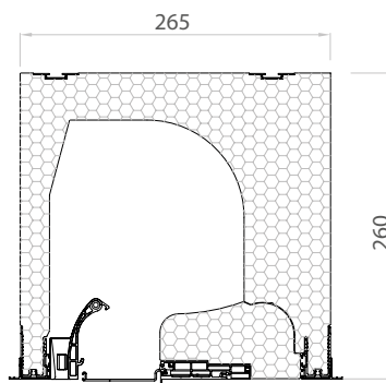
DK-RNT 260 Revisionsdeckel von außen
