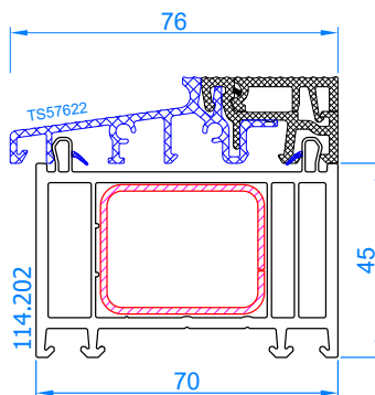
Verbreiterung 45mm Code: 114.202 Verbreiterungf unter einer niedrigen ALU-Schwelle (TS57622)
