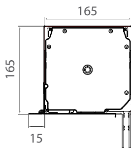
DK-RSP Kasten 165
