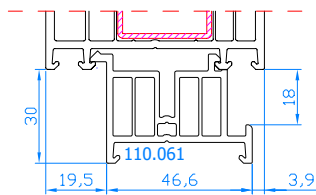
Fensterbankanschlußprofil 30x46,6 Code: 110.061
