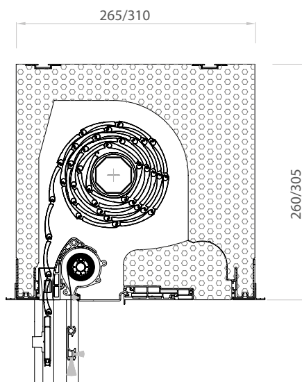
DK-RNT 260/305 Revisionsdeckel von außen
