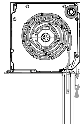
UNTERPUTZSYSTEM DK-RSP integriertes Insektenschutzgitter
