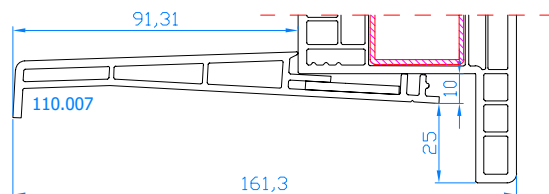
Fensterbankanschlußprofil für DPP-70 R35 Code: 110.007
