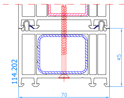
Verbreiterung 45mm Code: 114.202 für DPP-70
