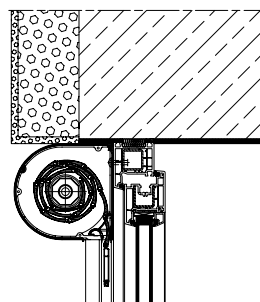
DK-RZO in der Nische montiert
