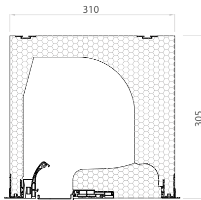
DK-RNT 305 Revisionsdeckel von außen
