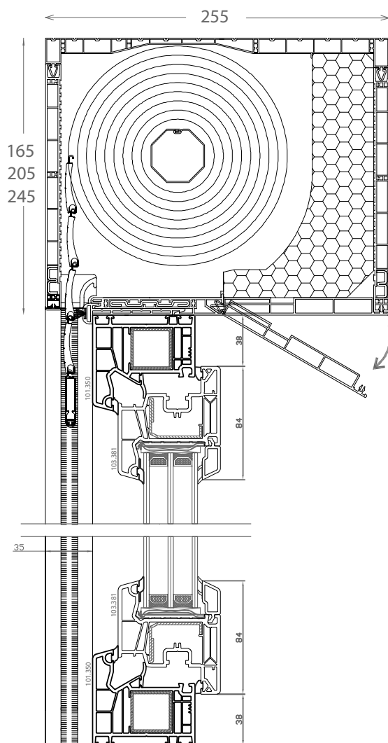
DPQ-76 Aufsatzrollladen: DK-RNB Querschnitt
