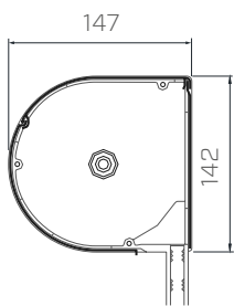
DK-RZO Kasten 137
