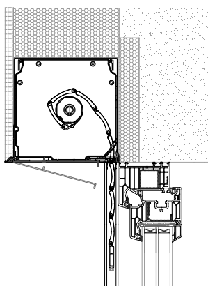
DK-RSP in der Nische montiert
