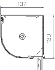
DK-RZP Kasten 137
