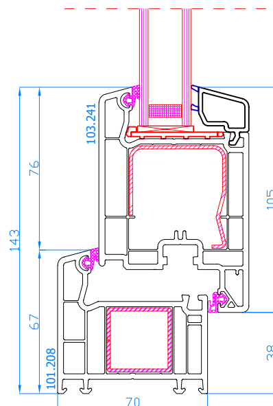
DPP-70 Breiter Flügel Rahmen: 101.208 Flügel: 103.241
