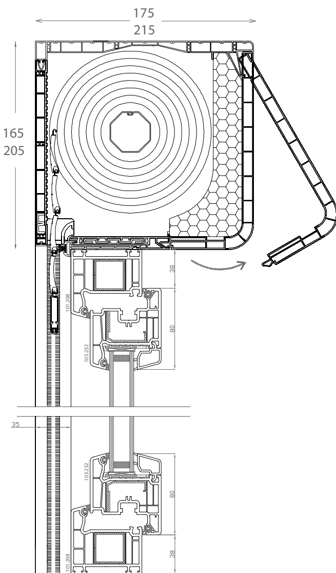
DPP-70 Aufsatzrollladen: DK-RNC Querschnitt
