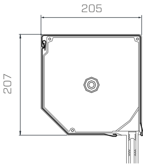
DK-RZS Kasten 205
