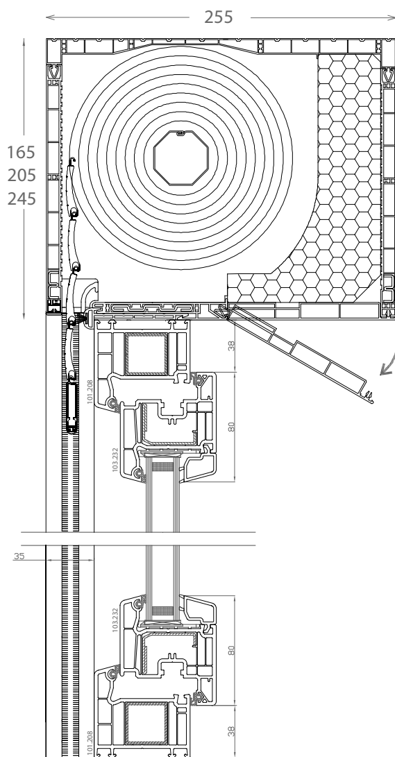
DPP-70 Aufsatzrollladen: DK-RNB Querschnitt
