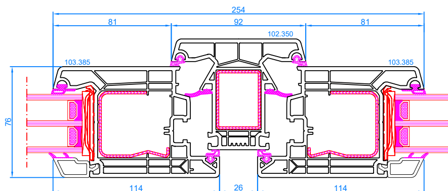
DPQ-76 Setzpfofen Setzpfofen: 102.350 breiter Flügel: 103.385
