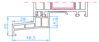
Fensterbankanschlußprofil 28x48,5 Code: 110.079
