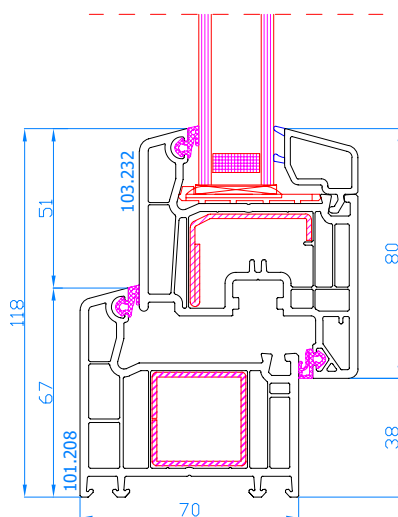
DPP-70 Standardflügel Rahmen: 101.208 Flügel: 103.232
