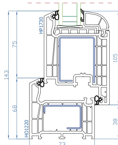
DPB-73 Breiter Flügel Rahmen: HO1220 breiter Flügel: HP1730
