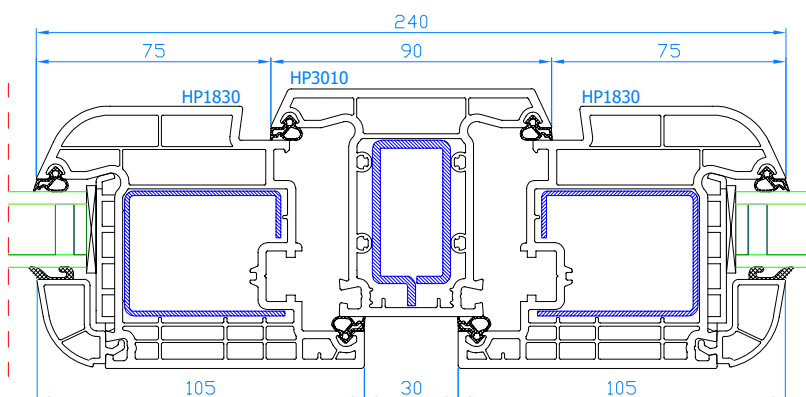
DPB-73+ Setzpfosten Setzpfosten: HP3010 breiter Flügel: HP1830
