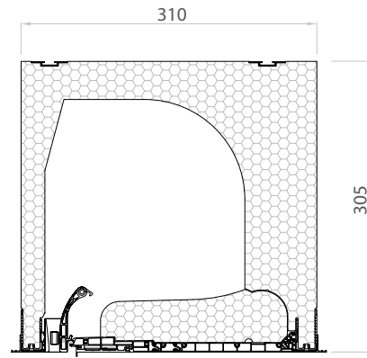
DK-RNT 305 Revisionsdeckel von innen
