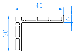
Abdeckwinkel 30x40 Code: 109.070
