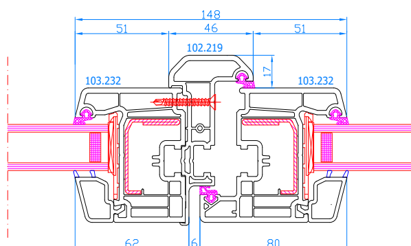
DPP-70 Stulp Stulp: 102.219 Flügel: 103.232
