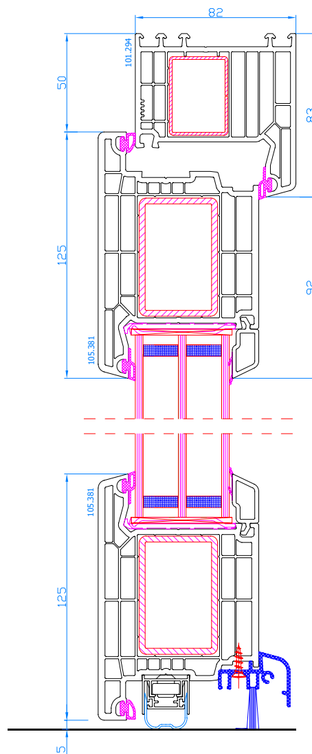
DPQ-82 Eingangstür mit absenkbarer Leiste (ohne Schwelle) nach außen öffnend Rahmen: 101.294 Flügel: 105.381
