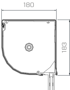
DK-RZP Kasten 180
