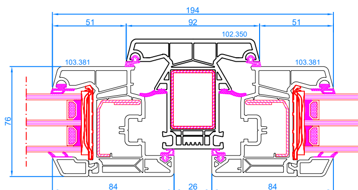
DPQ-76 Setzpfofen Setzpfofen: 102.350 Flügel: 103.381
