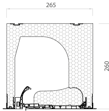
DK-RNT 260 Revisionsdeckel von innen
