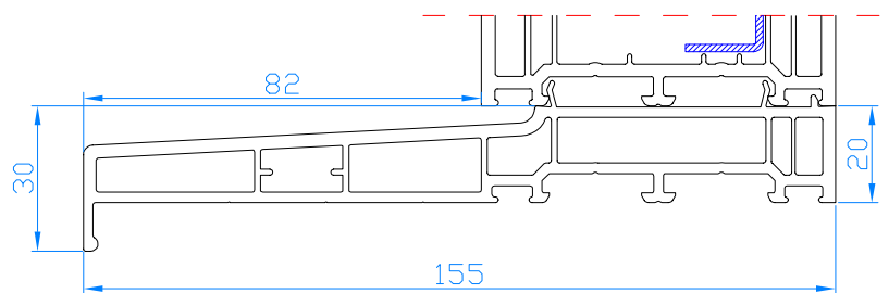
Fensterbankanschlußprofil 155x20
