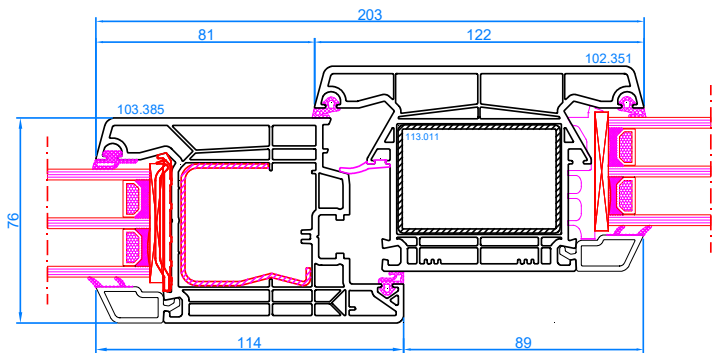
DPQ-76 Setzpfosten Setzpfosten: 102.351 breiter Flügel: 103.385
