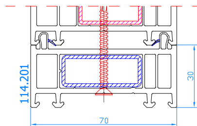
Verbreiterung 30mm Code: 114.201 für DPP-70
