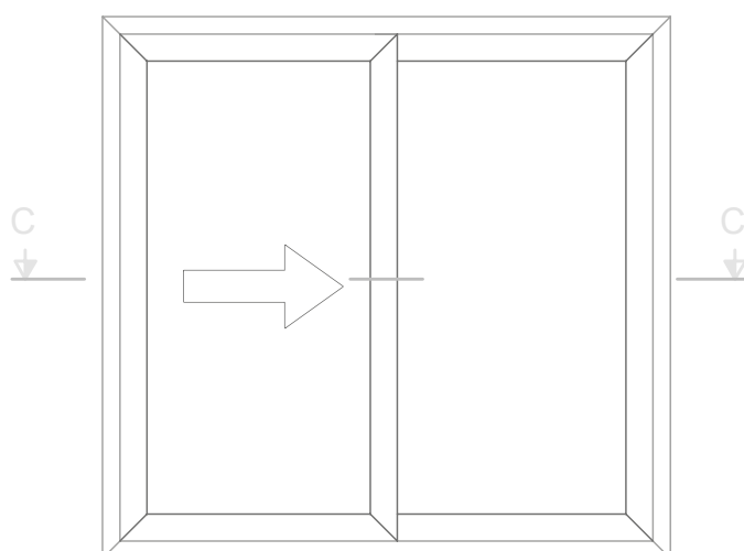
DPQ-82AL HST Öffnungsschema Schema A
