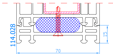
Verbreiterung 15mm Code: 114.028 für DPP-70
