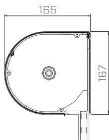
DK-RZO Kasten 165
