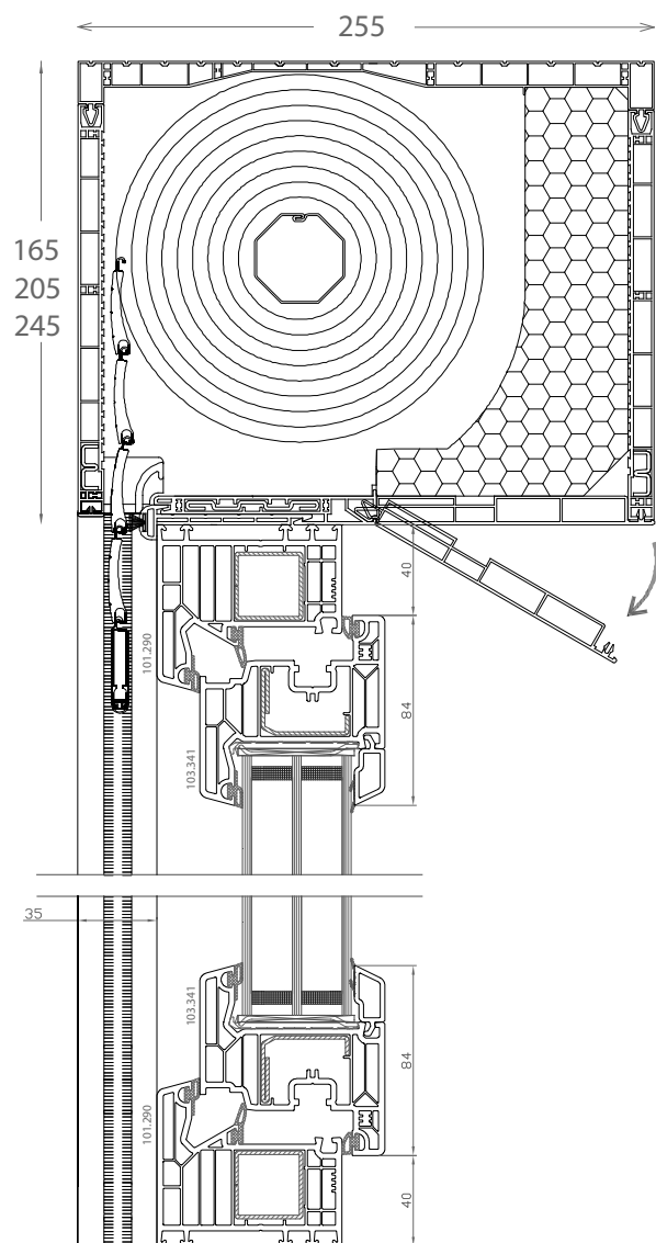
DPQ-82 Aufsatzrollladen: DK-RNB Querschnitt
