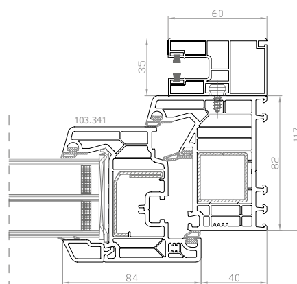
DPQ-82 Draufsicht
