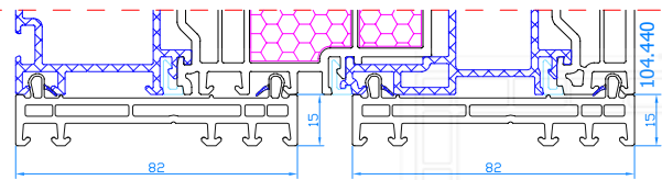
2x Verbreiterung 15mm Code: 114.040 für HST DPQ-82
