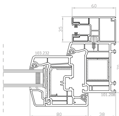
DPP-70 Aufsatzrollladen: DK-RNB Querschnitt
