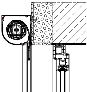
DK-RZP vorne an der Wand montiert
