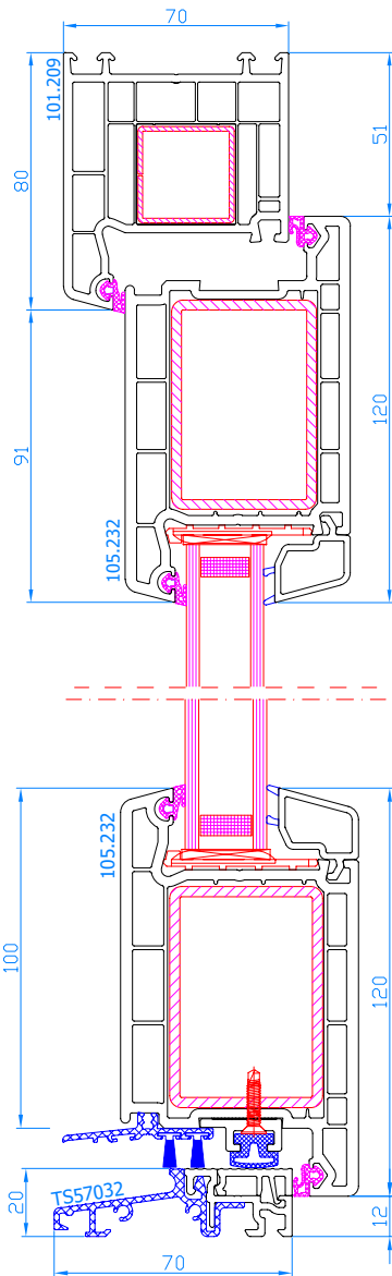
DPP-70 Eingangstür mit niedriger ALU-Schwelle nach innen öffnend ALU-Schwelle: TS57032 Rahmen: 101.209 Flügel: 105.232
