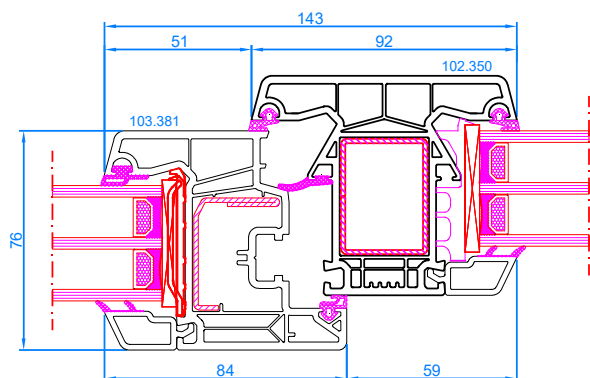
DPQ-76 Setzpfofen Setzpfofen: 102.350 Flügel: 103.381
