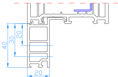
Fensterbankanschlußprofil 40x20
