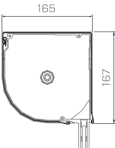
DK-RZP Kasten 165
