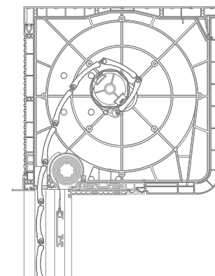
AUFSATZSYSTEM DK-RNC integriertes Insektenschutzgitter
