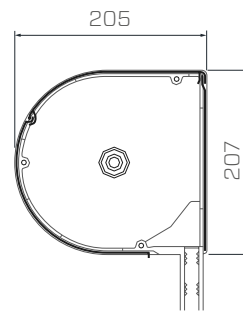
DK-RZO Kasten 205
