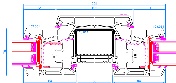
DPQ-76 Setzpfosten Setzpfosten: 102.351 Flügel: 103.381
