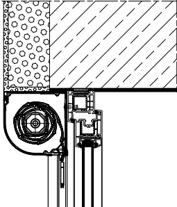
DK-RZP in der Nische montiert
