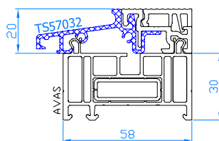
Transportleiste für niedrige ALU-Schwelle (TS57032) Code: AVAS02
