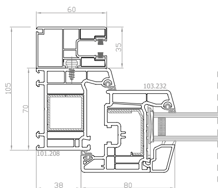
DPP-70 Aufsatzrollladen: DK-RNC Querschnitt
