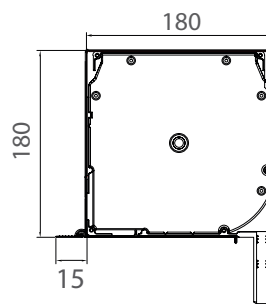
DK-RSP Kasten 180
