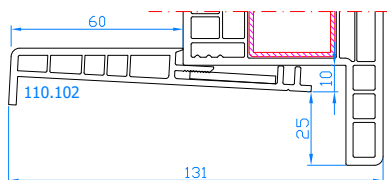
Fensterbankanschlußprofil für DPP-70 R35 Code: 110.102
