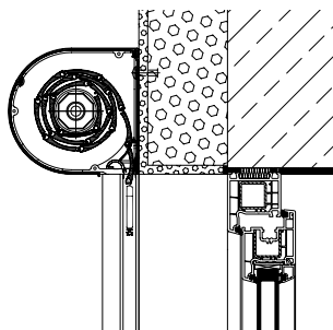
DK-RZO vorne an der Wand montiert
