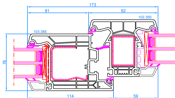
DPQ-76 Setzpfofen Setzpfofen: 102.350 breiter Flügel: 103.385
