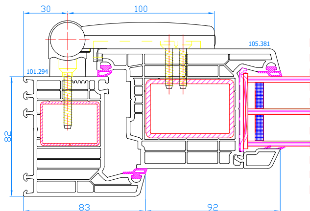
DPQ-82 Eingangstür nach außen öffnend (Draufsicht) Rahmen: 101.294 Flügel: 105.381
