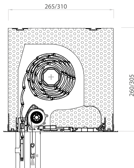
DK-RNT 260/305 Revisionsdeckel von innen
