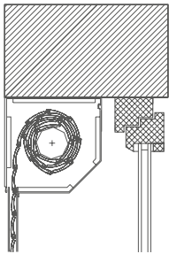
DK-RZS in der Nische montiert
