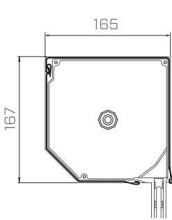
DK-RZS Kasten 165
