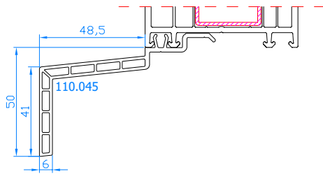
Fensterbankanschlußprofil 50x48,5 Code: 110.045
