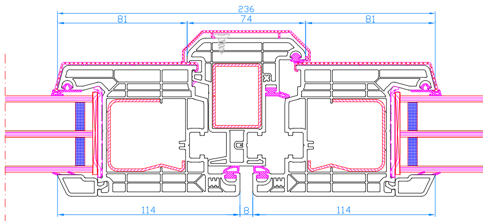
DPQ-82 AL Stulp Stulp: 102.316 breiter Flügel: 103.345
