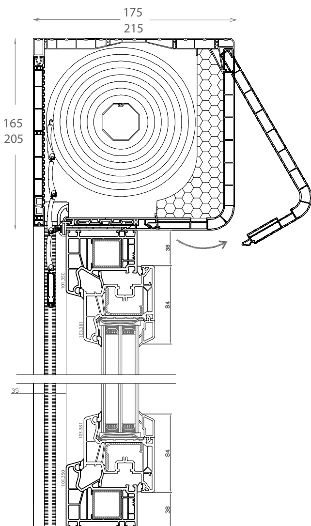
DPQ-76 Aufsatzrollladen: DK-RNC Querschnitt
