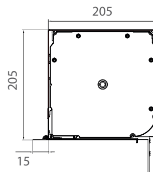
DK-RSP Kasten 205
