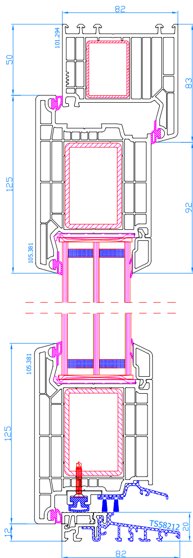
DPQ-82 Eingangstür mit niedriger ALU-Schwelle nach außen öffnend ALU-Schwelle: 104.460 Rahmen: 101.294 Flügel: 105.381
