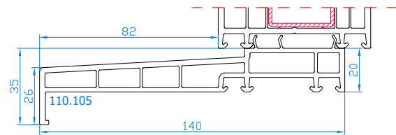
Fensterbankanschlußprofil 20x140 Code: 110.105
