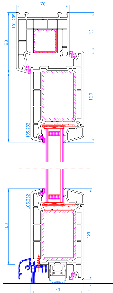
DPP-70 Eingangstür mit absenkbarer Leiste (ohne Schwelle) nach innen öffnend Rahmen: 101.209 Flügel: 105.232
