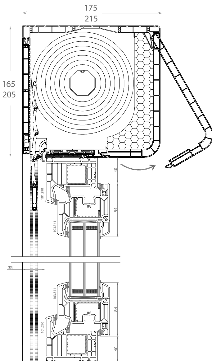
DPQ-82 Aufsatzrollladen: DK-RNC Querschnitt
