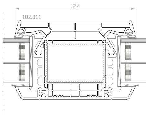
DPQ-82 Montante fisso montante: 102.311
