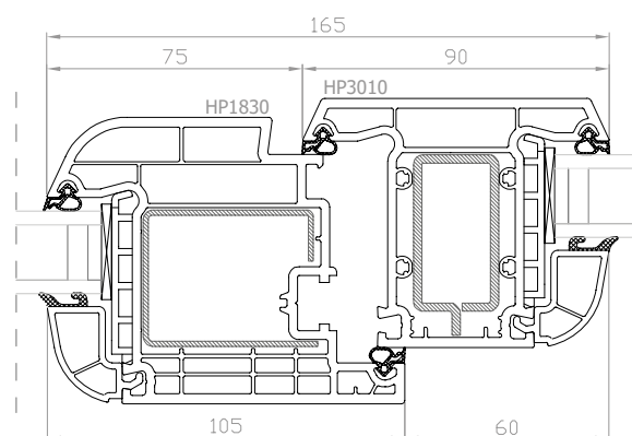
DPB-73+ Finestra apribile con montante fisso, anta maggiorata
