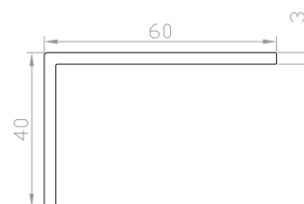
Coprifilo angolare 60x40
