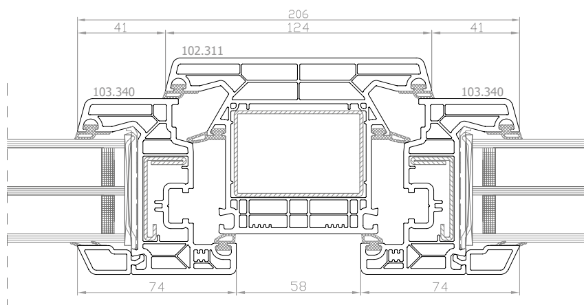
DPQ-82 Lumia Line Finestra a 2 ante con montante fisso, anta ridotta
