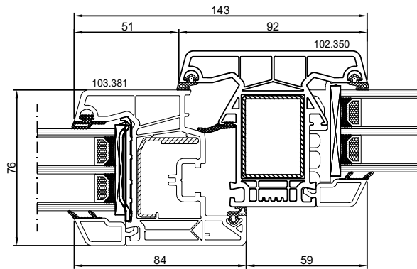
DPQ-76 Finestra con montante fisso
