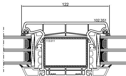
DPQ-76 Montante fisso Montante: 102.351
