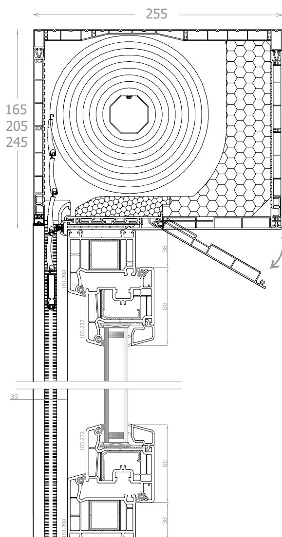
DPP-70 avvolgibile monoblocco: DK-RNB sezione verticale
