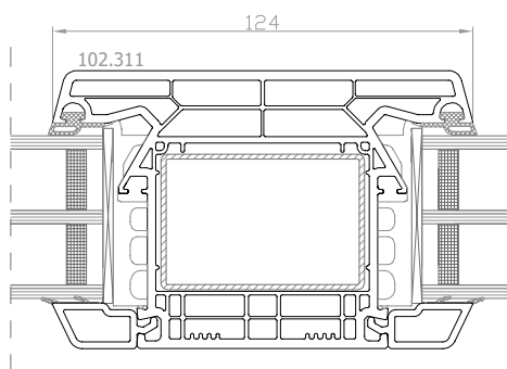
DPQ-82 Montante fisso montante: 102.311
