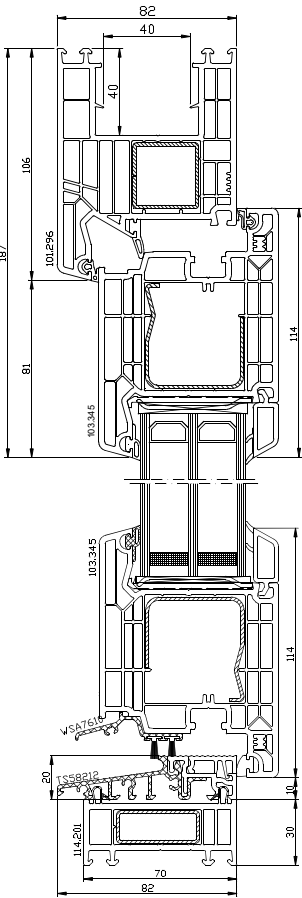
DPQ-82 H Anta 114 Soglia in alluminio
