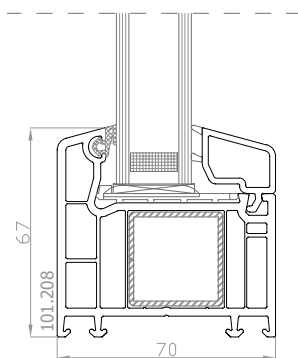
DPP-70 Finestra fissa
