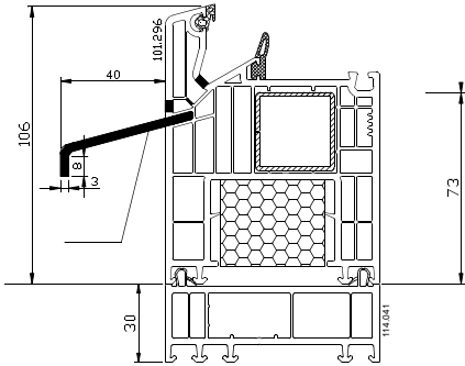
DPQ-82 H Davanzale in alluminio Isolamento termico
