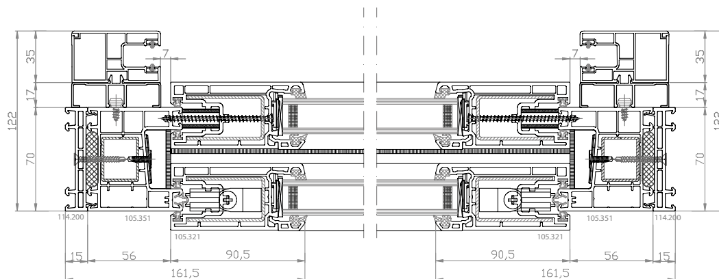
EKOSOL sezione orizzontale
