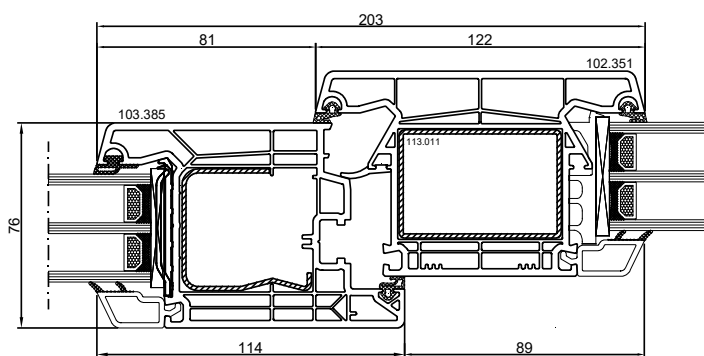
DPQ-76 Finestra con montante fisso
