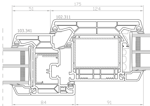
DPQ-82 Finestra con montante fisso
