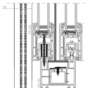
EKOSOL avvolgibile monoblocco: DK-RNB sezione verticale
