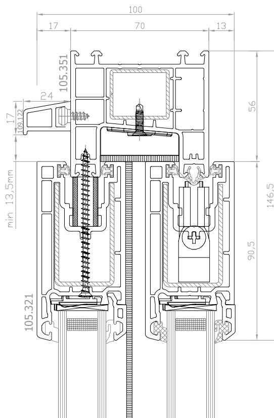
EKOSOL Schiebetur Sezione superiore
