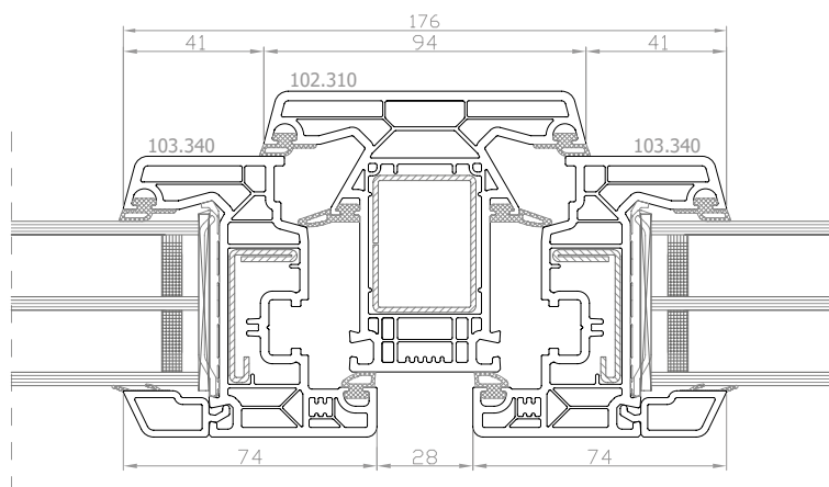
DPQ-82 Lumia Line Finestra a 2 ante con montante fisso, anta ridotta
