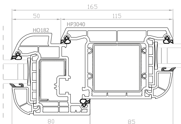
DPB-73+ Finestra apribile con montante fisso
