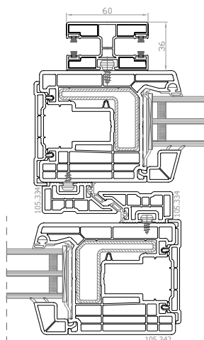
DPP-82 HST avvolgibile monoblocco: DK-RNB sezione orizzontale
