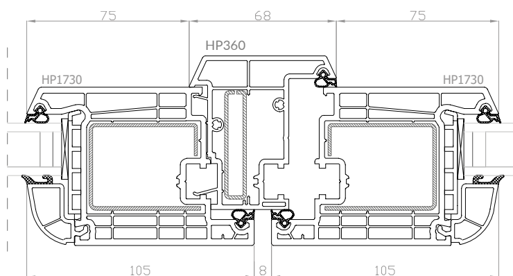
DPB-73 Finestra a 2 ante con montante mobile, anta maggiorata
