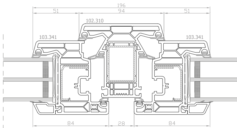
DPQ-82 Finestra a 2 ante con montante fisso
