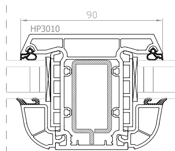
DPB-73+ Montante fisso montante: HP3010
