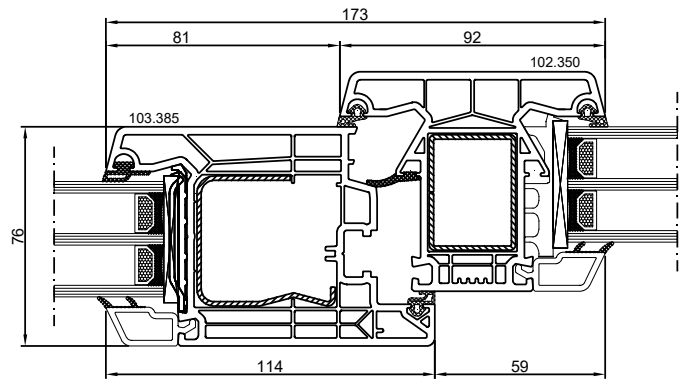
DPQ-76 Finestra con montante fisso, anta maggiorata.
