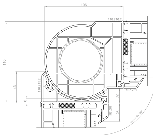
116.229 connettore ad angolo 90°
