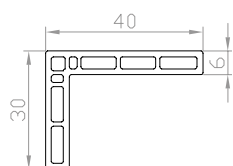
Coprifilo angolare perforato 30x40
