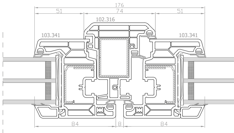
DPQ-82 Finestra a 2 ante con montante mobile
