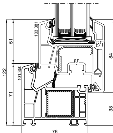
DPQ-76 Finestra apribile
