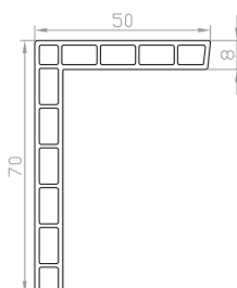
Coprifilo angolare perforato 50x70
