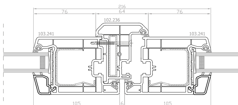
DPP-70 Finestra a 2 ante con montante mobile, anta maggiorata
