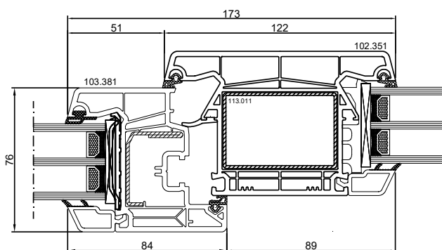
DPQ-76 Finestra con montante fisso
