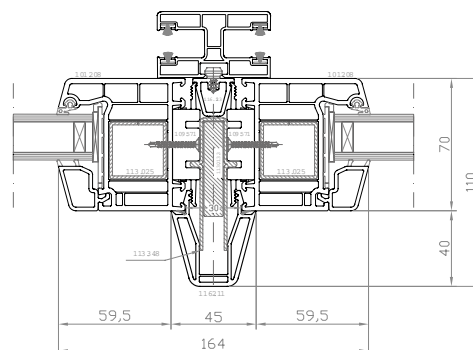
116.213/211, sotto la tapparella
