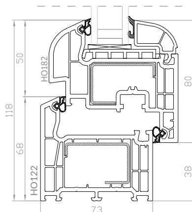
DPB-73+ Finestra apribile
