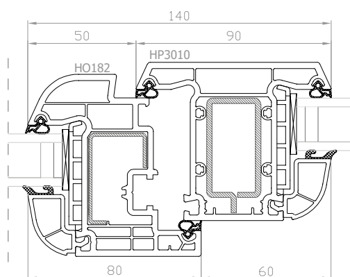
DPB-73+ Finestra apribile con montante fisso
