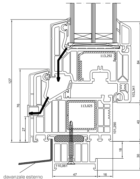
DPQ-82 AL Fori di drenaggio (frontale)
