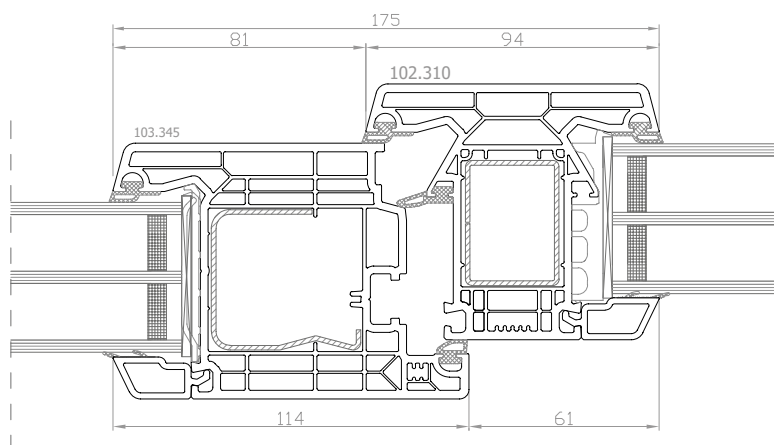
DPQ-82 Montante fisso montante: 102.310
