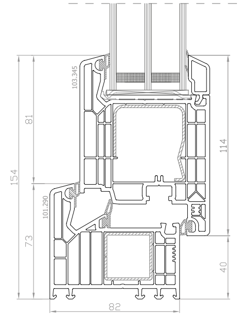
DPQ-82 Finestra apribile, anta maggiorata
