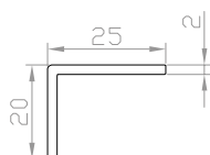
Coprifilo angolare 25x20
