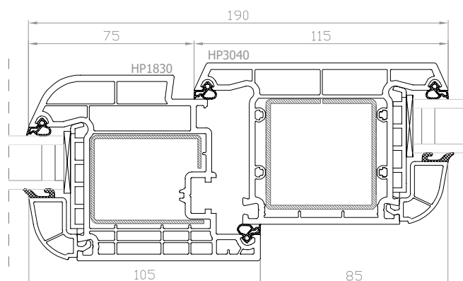
DPB-73+ Finestra apribile con montante fisso, anta maggiorata
