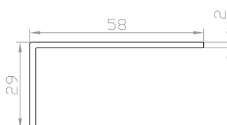
Coprifilo angolare 58x29
