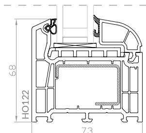
DPB-73+ Finestra fissa
