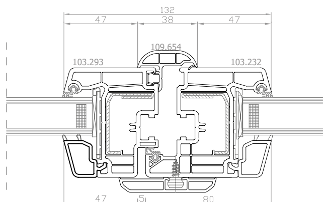
DPP-70 Finestra a 2 ante con montante mobile, maniglia centrale
