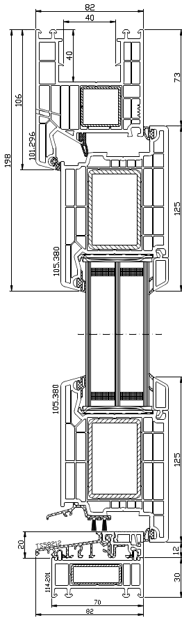
DPQ-82 H Porta d'ingresso con apertura verso l'interno
