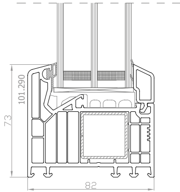
DPQ-82 Finestra fissa
