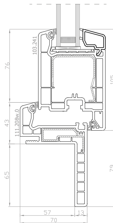
DPP-70 R65 Finestra apribile, profilo restauro R65, anta maggiorata
