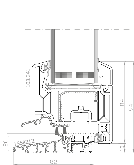
DPQ-82 Porta finestra soglia bassa in allu, apertura verso l'interno
