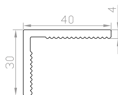
Coprifilo angolare 40x30
