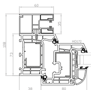
DPB-73 sezione orizzontale
