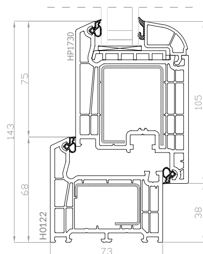
DPB-73 Finestra apribile, anta maggiorata
