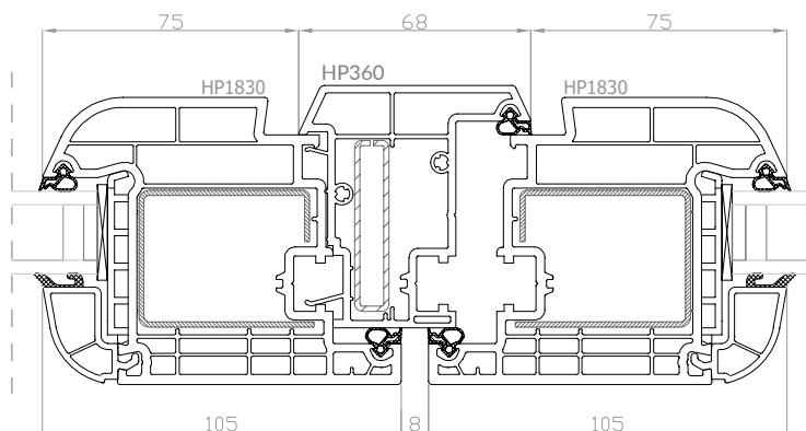
DPB-73+ Finestra a 2 ante con montante mobile, anta maggiorata
