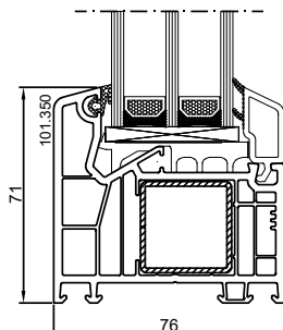
DPQ-76 Finestra fissa nel telaio Telaio: 101.350
