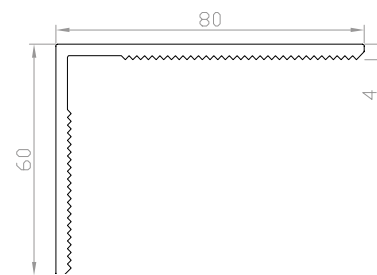
Coprifilo angolare 80x60
