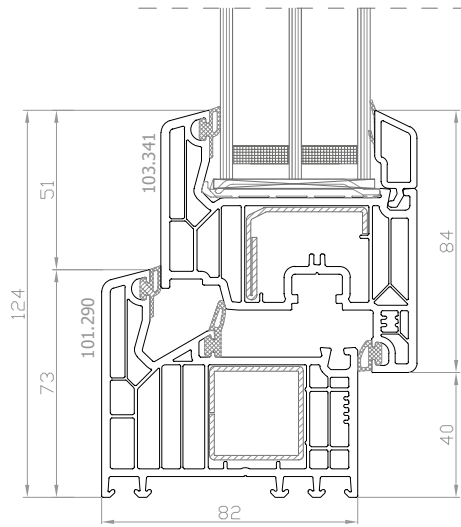
DPQ-82 Finestra apribile
