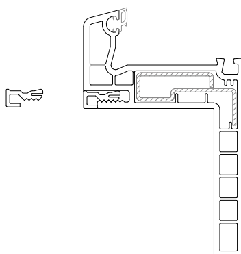
DPP-70 R65 Profilo di riempimento 111.033
