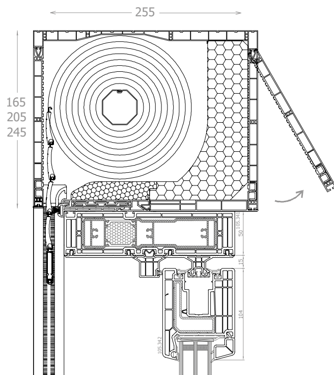
DPQ-82 HST avvolgibile monoblocco: DK-RNB sezione verticale
