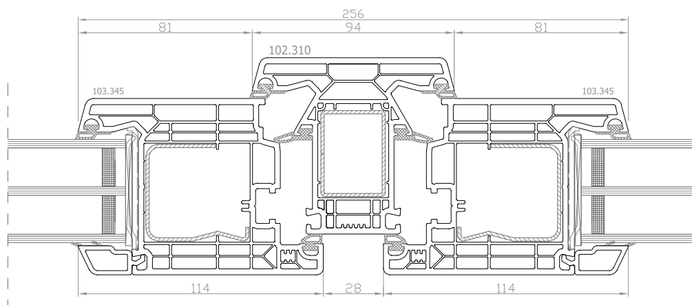
DPQ-82 Finestra a 2 ante con montante fisso, anta maggiorata
