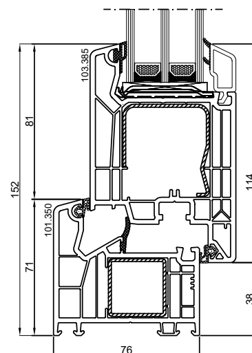
DPQ-76 Finestra apribile con anta maggiorata
