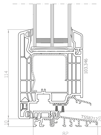
DPQ-82 Porta finestra soglia bassa in allu, apertura verso l'esterno
