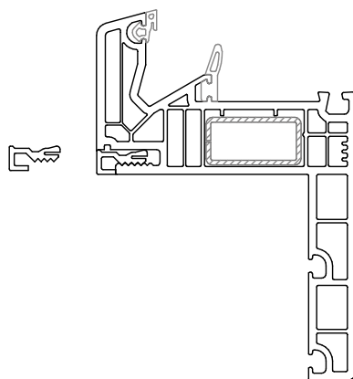
DPQ-82 R65 Profilo di riempimento 111.033
