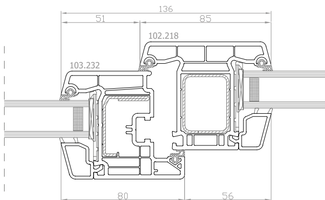
DPP-70 Finestra con montante fisso
