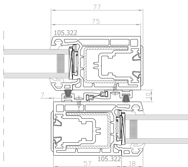
EKOSOL Schiebefenster Sezione laterale
