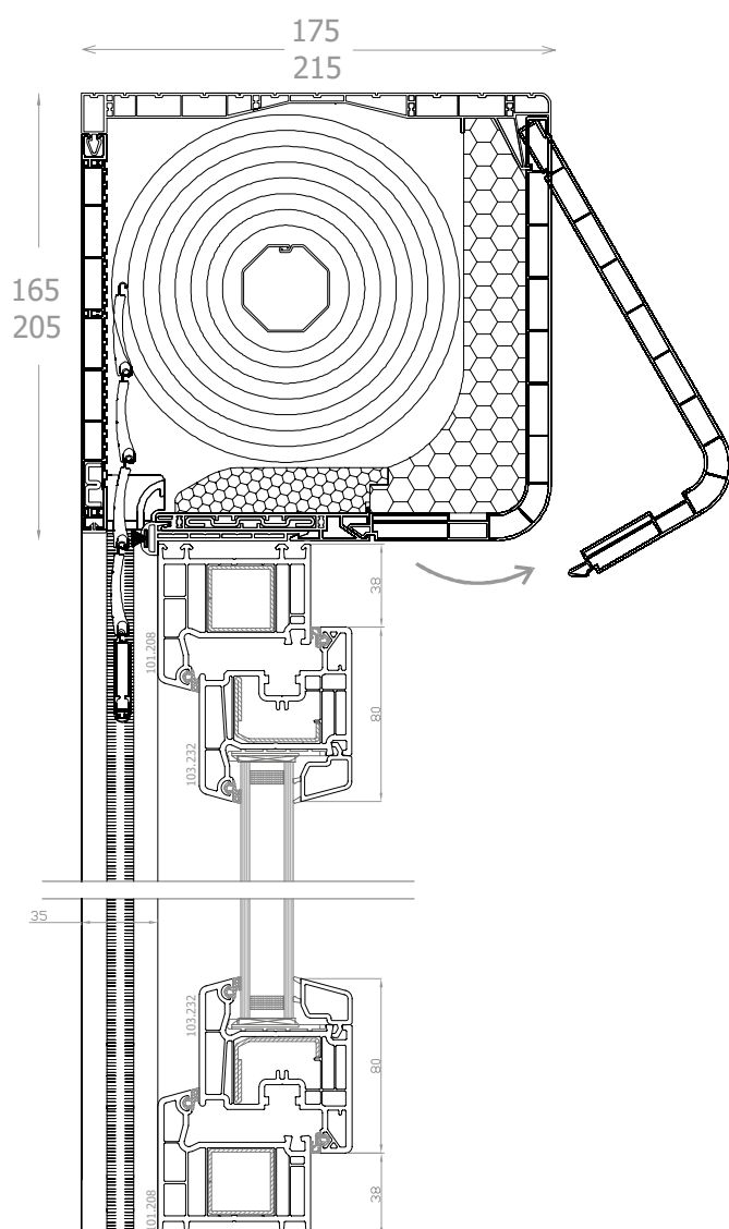
DPP-70 avvolgibile monoblocco: DK-RNC sezione verticale
