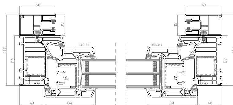
DPQ-82 sezione orizzontale
