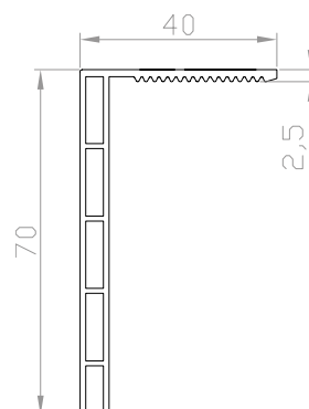
Coprifilo angolare perforato 40x70
