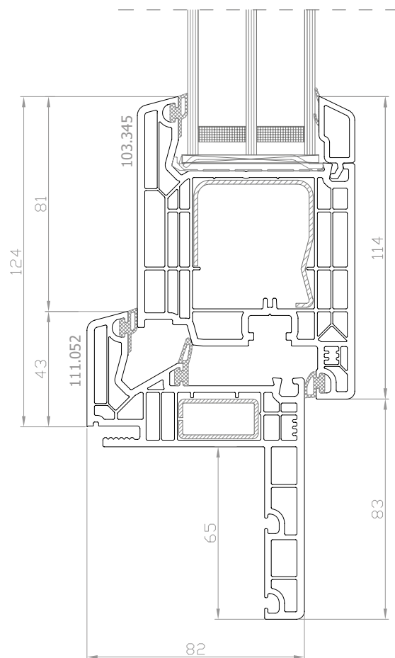
DPQ-82 R65 Finestra apribile, profilo restauro R65, anta maggiorata
