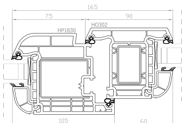
DPB-73+ Finestra con montante fisso, anta maggiorata
