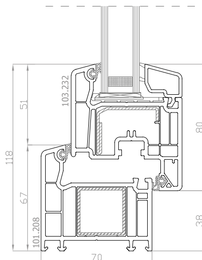
DPP-70 Finestra apribile
