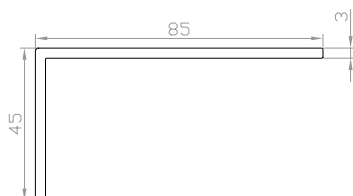
Coprifilo angolare 85x45
