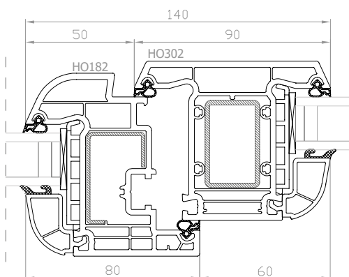
DPB-73+ Finestra con montante fisso
