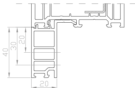
Aletta a scatto 40x20
