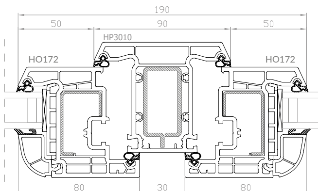
DPB-73 Finestra a 2 ante con montante fisso
