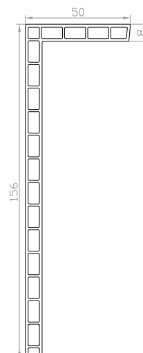
Coprifilo angolare perforato 50x156
