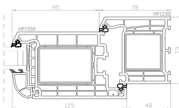
DPB-73 Porta d'ingresso, apertura verso l'interno (sezione orizzontale)
