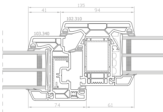
DPQ-82 Lumia Line Finestra con montante fisso, anta ridotta
