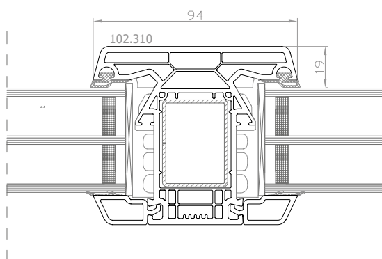
DPQ-82 Montante fisso montante: 102.310
