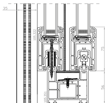
EKOSOL avvolgibile monoblocco: DK-RNC sezione verticale
