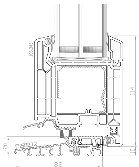
DPQ-82 Porta finestra soglia bassa in allu, anta maggiorata, apertura verso l'interno
