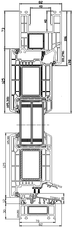
DPQ-82 H Porta d'ingresso con apertura verso l'esterno
