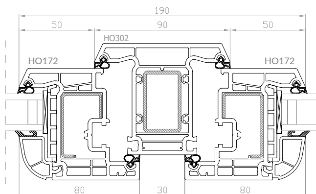
DPB-73 Finestra a 2 ante con montante fisso
