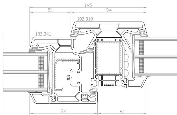
DPQ-82 Finestra con montante fisso
