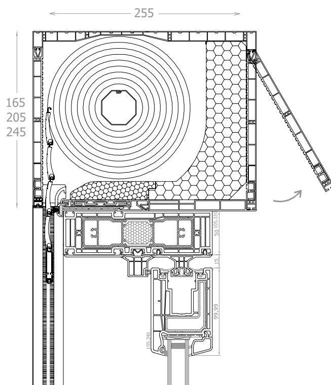
DPP-70 HST avvolgibile monoblocco: DK-RNB sezione verticale
