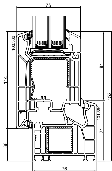
DPQ-76 Anta con apertura verso esterno, anta maggiorata
