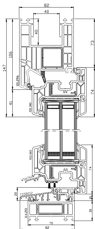
DPQ-82 H Anta 74mm Soglia in alluminio
