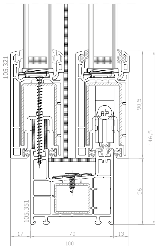
EKOSOL Schiebetur Sezione inferiore
