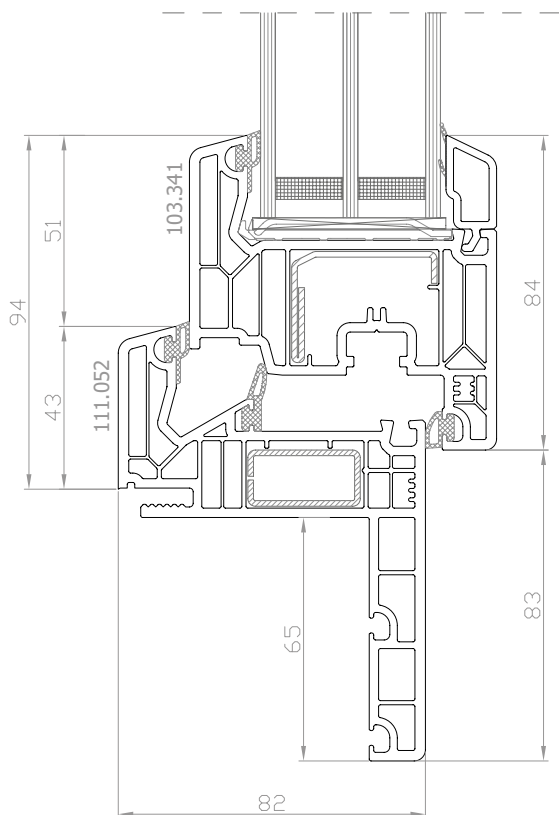
DPQ-82 R65 Finestra apribile, profilo restauro R65
