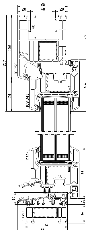
DPQ-82 H Soglia in alluminio
