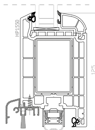
DPB-73 Porta d'ingresso senza soglia, apertura verso l'interno, barra parafreddo
