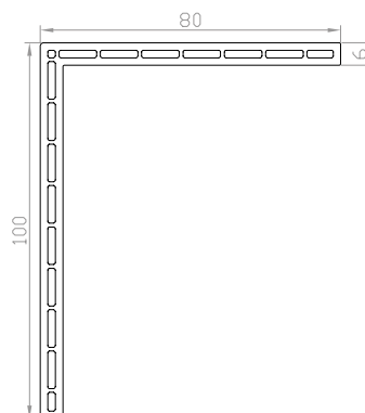
Coprifilo angolare perforato 80x100
