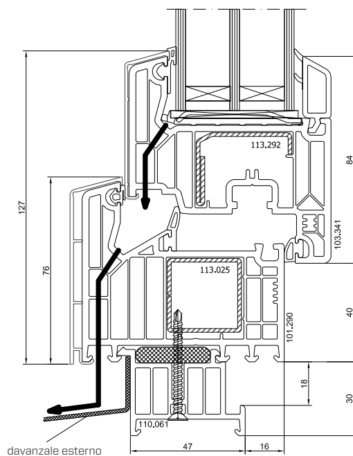
DPQ-82 AL Fori di drenaggio nascosti (lato inferiore)
