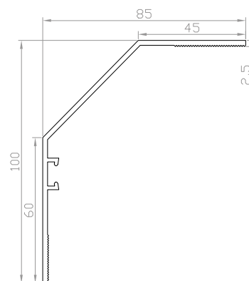
Coprifilo angolare pan coupe 85x100
