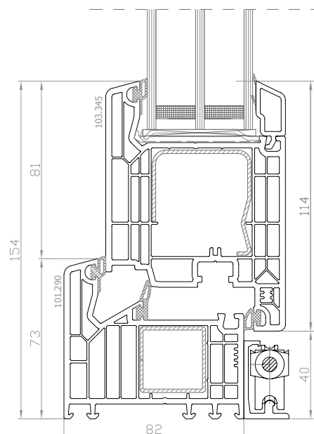
DPQ-82 Traslante-scorrevole H > 2,2 m
