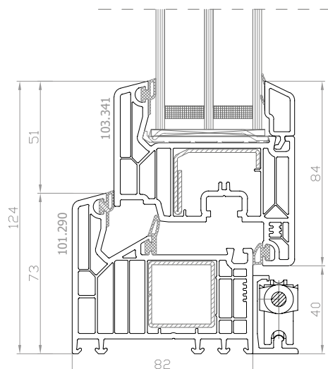
DPQ-82 Traslante-scorrevole H < 2,2 m
