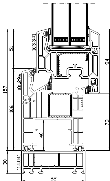
DPQ-82 H Anta 84mm
