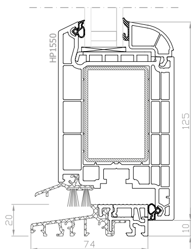
DPB-73 Porta d'ingresso con soglia bassa in allu, apertura verso l'interno
