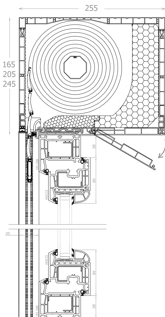
DPB-73 avvolgibile monoblocco: DK-RNC sezione verticale
