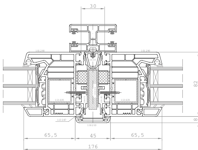
116.213/210, sotto la tapparella
