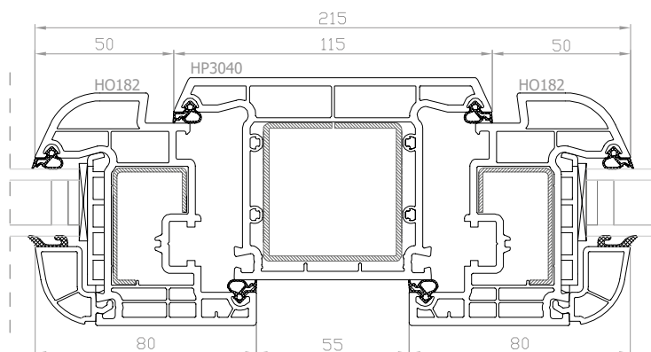
DPB-73+ Finestra a 2 ante con montante fisso
