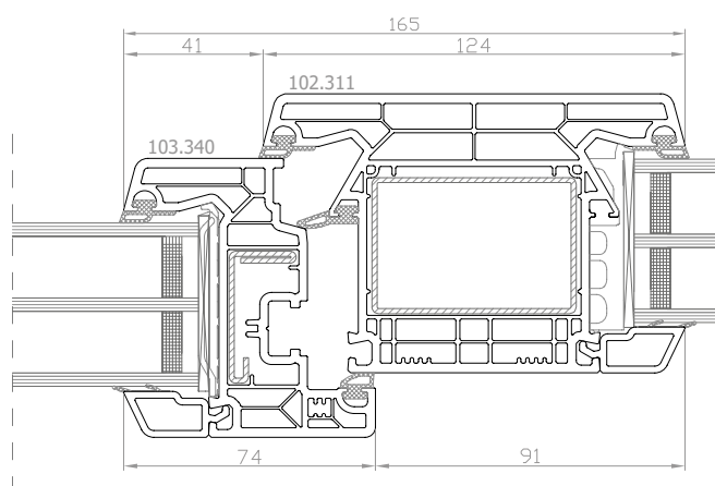
DPQ-82 Lumia Line Finestra con montante fisso, anta ridotta
