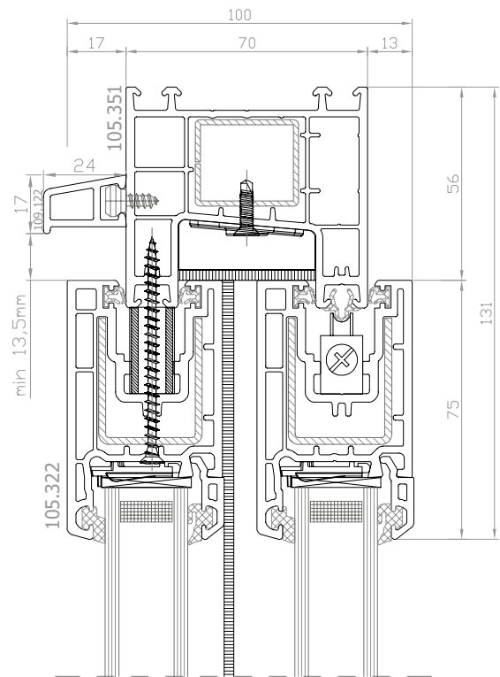
EKOSOL Schiebefenster Sezione superiore
