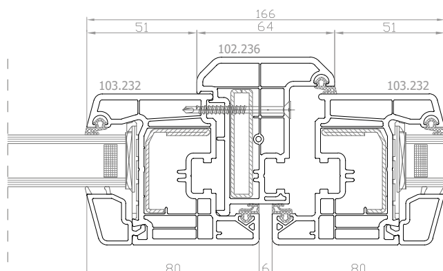
DPP-70 Finestra a 2 ante con montante mobile
