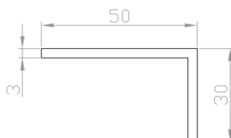
Coprifilo angolare 50x30
