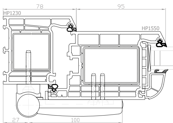
DPB-73 Porta d'ingresso, apertura verso l'interno (sezione orizzontale)
