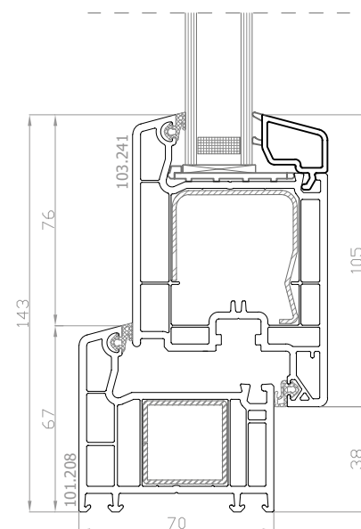
DPP-70 Finestra apribile con anta maggiorata
