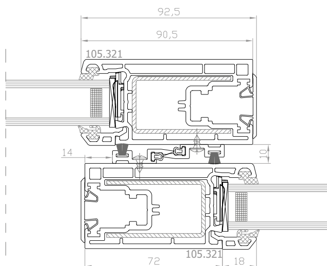
EKOSOL Schiebetur Sezione laterale
