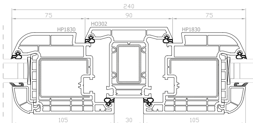
DPB-73+ Finestra a 2 ante con montante fisso, anta maggiorata
