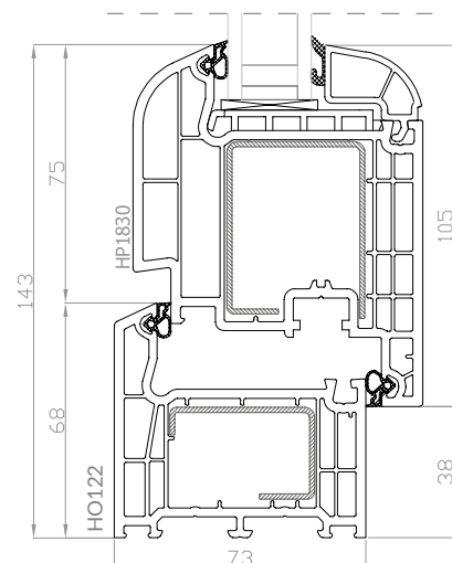
DPB-73+ Finestra apribile con anta maggiorata
