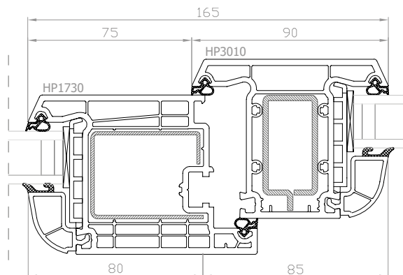
DPB-73 Finestra con montante fisso, anta maggiorata
