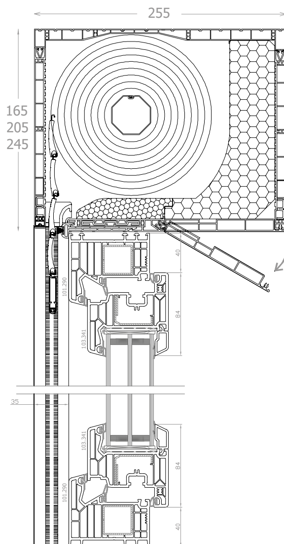
DPQ-82 avvolgibile monoblocco: DK-RNB sezione verticale
