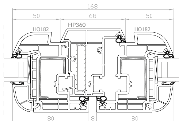
DPB-73+ Finestra a 2 ante con montante mobile
