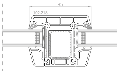
DPP-70 Montante fisso montante: 102.218
