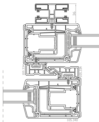
DPP-70 HST avvolgibile monoblocco: DK-RNB sezione orizzontale
