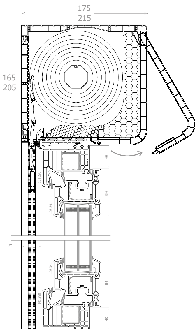
DPQ-82 avvolgibile monoblocco: DK-RNC sezione verticale
