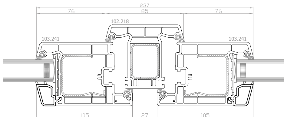
DPP-70 Finestra a 2 ante con montante fisso, anta maggiorata
