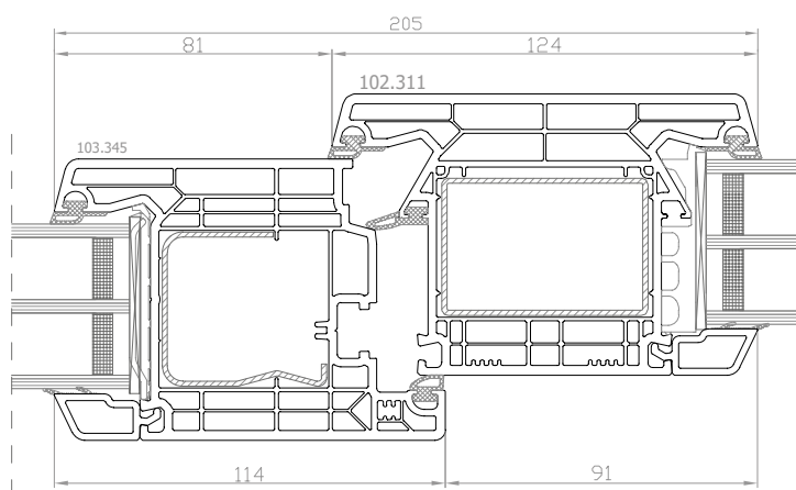
DPQ-82 Montante fisso montante: 102.311
