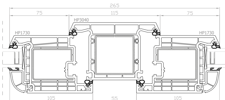
DPB-73 Finestra a 2 ante con montante fisso, anta maggiorata
