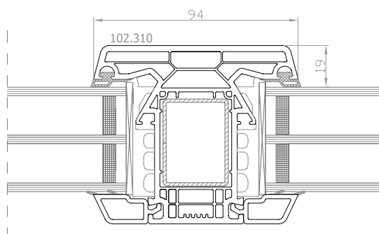
DPQ-82 Montante fisso montante: 102.310
