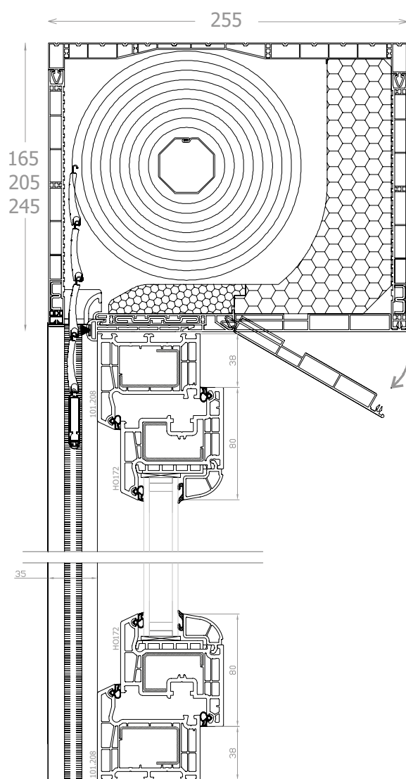
DPB-73 avvolgibile monoblocco: DK-RNB sezione verticale
