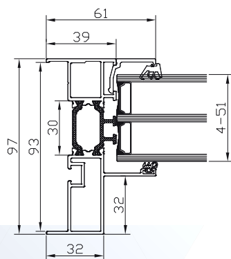
DA-65EF.M FW.06 (MONOBLOC 100)
