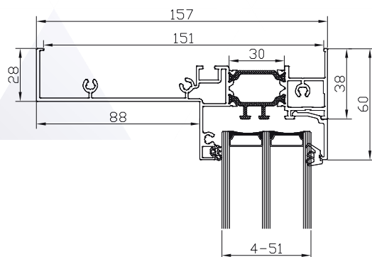
DA-65EF.M FW.04 (MONOBLOC 160)
