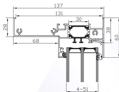
DA-65EF.M FW.03 (MONOBLOC 140)
