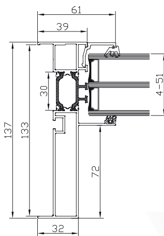
DA-65EF.M FW.08 (MONOBLOC 140)
