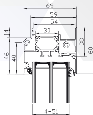
DA-65EF.M FW.05 (ONDER EEN ROLLUIK)
