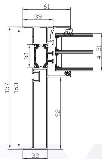
DA-65EF.M FW.09 (MONOBLOC 160)
