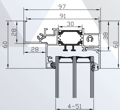
DA-65EF.M FW.01 (MONOBLOC 100)
