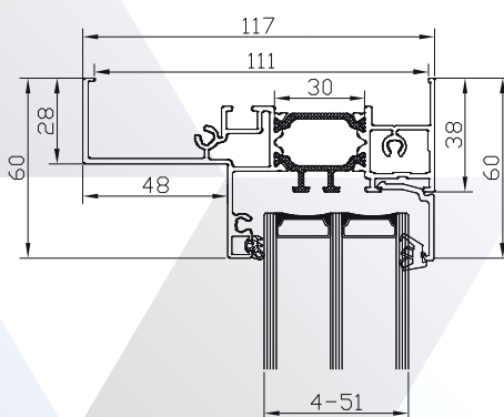
DA-65EF.M FW.02 (MONOBLOC 120)
