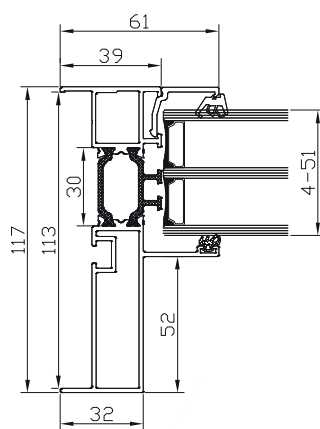
DA-65EF.M FW.07 (MONOBLOC 120)
